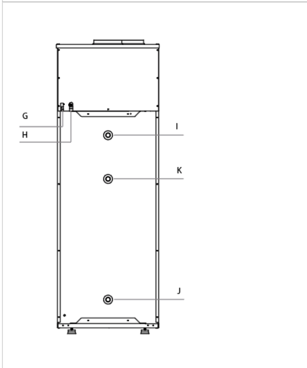
Figura 3. Conexiones traseras
