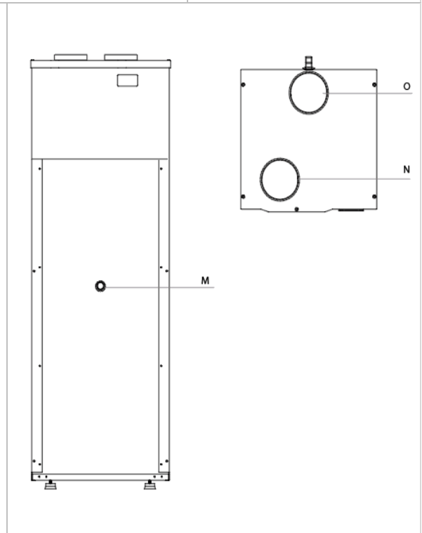
Figura 4. Conexiones delanteras
